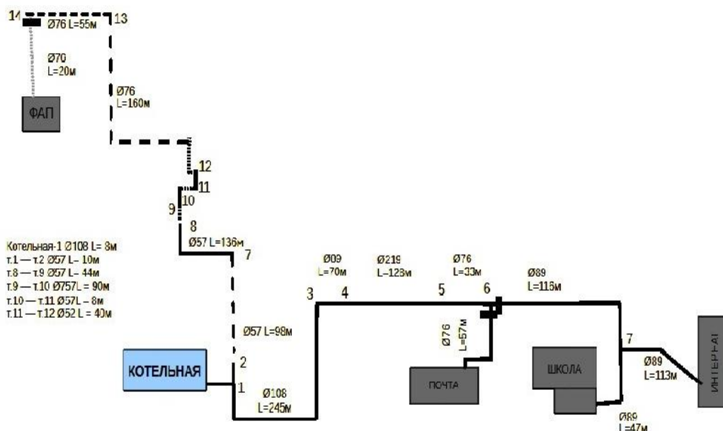
Рисунок 1.1. Общая схема теплоснабжения с. Колшево
